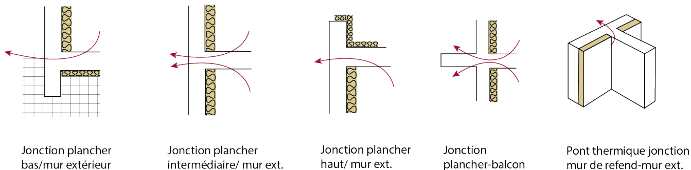
Figure 10 : Ponts thermiques les plus courants
