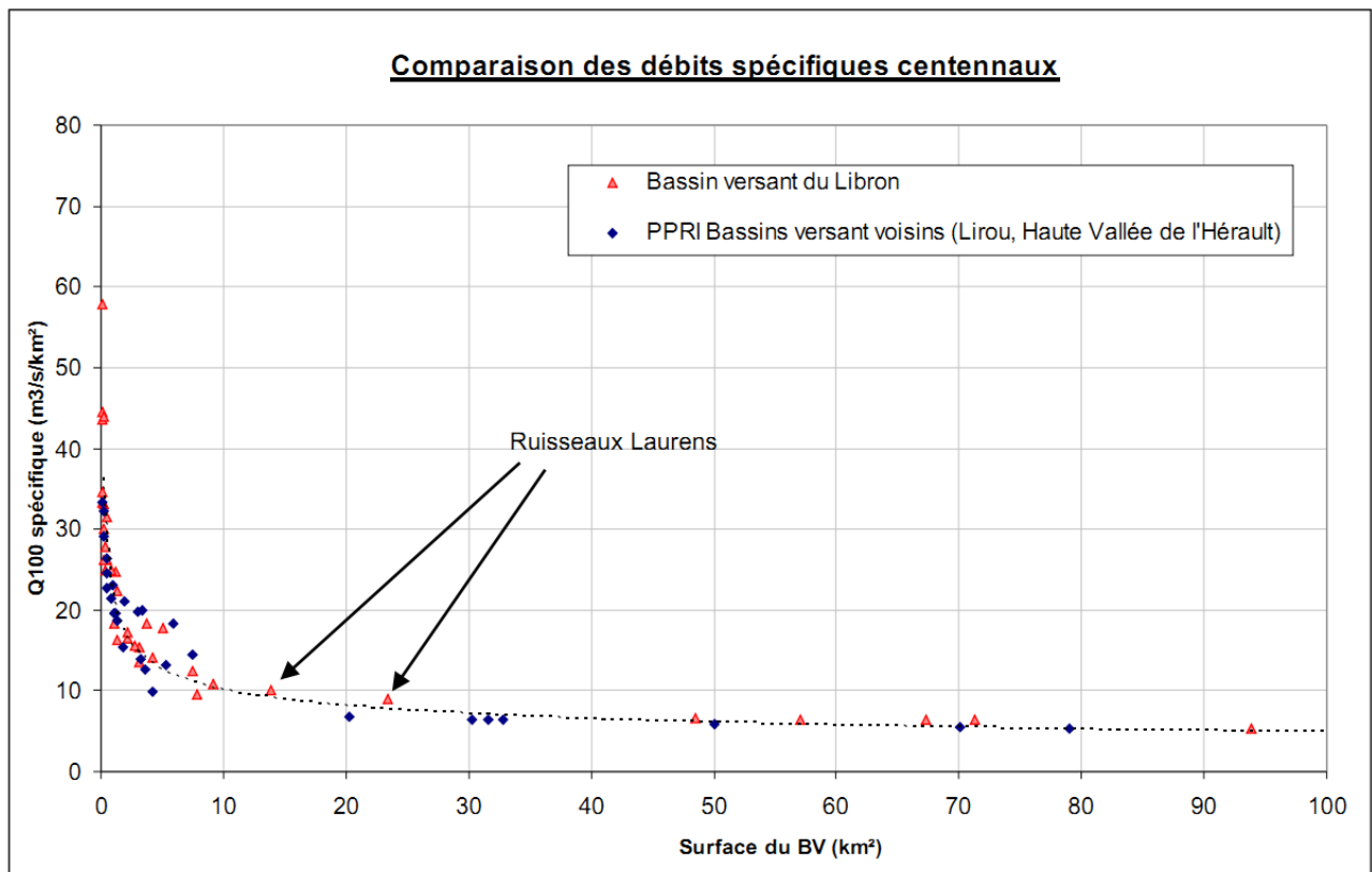
Débits centennaux spécifiques pour les bassins versants du Libron et du ruisseau de Naubine
