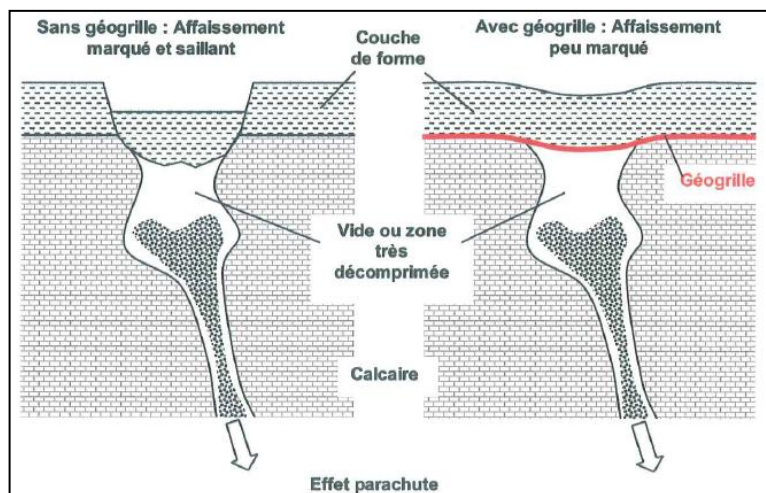
Figure 31 : « Effet parachute » d'une géogrille en prévention du risque de cavités souterraines [Source : ARCADIS]
